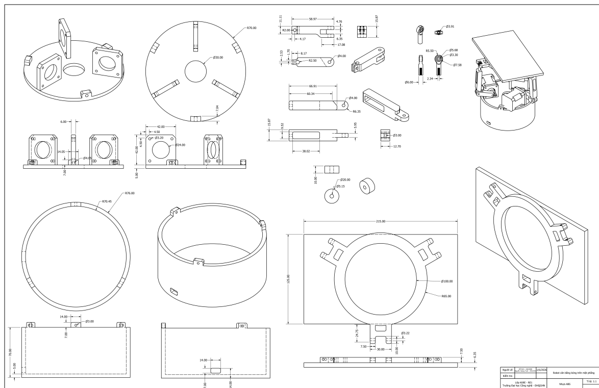
Hình 3.12: Bản vẽ kỹ thuật
