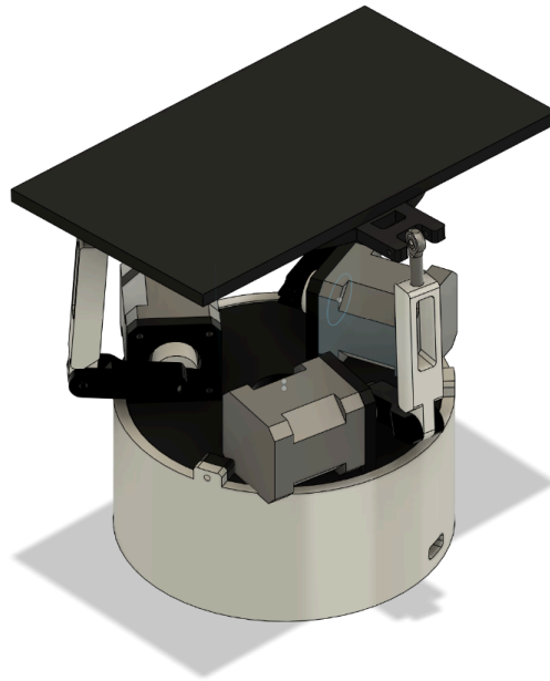
Hình 3.11: Mô hình 3D thiết kế cơ khí
